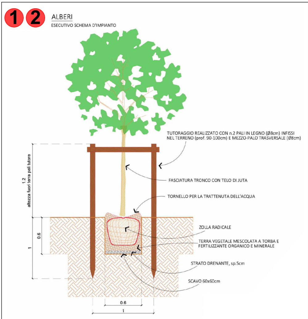
Particolare 1 (Particolare di messa a dimora)
